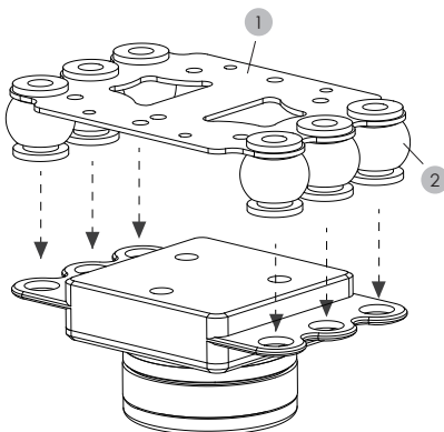
Damping Ball 减震球
